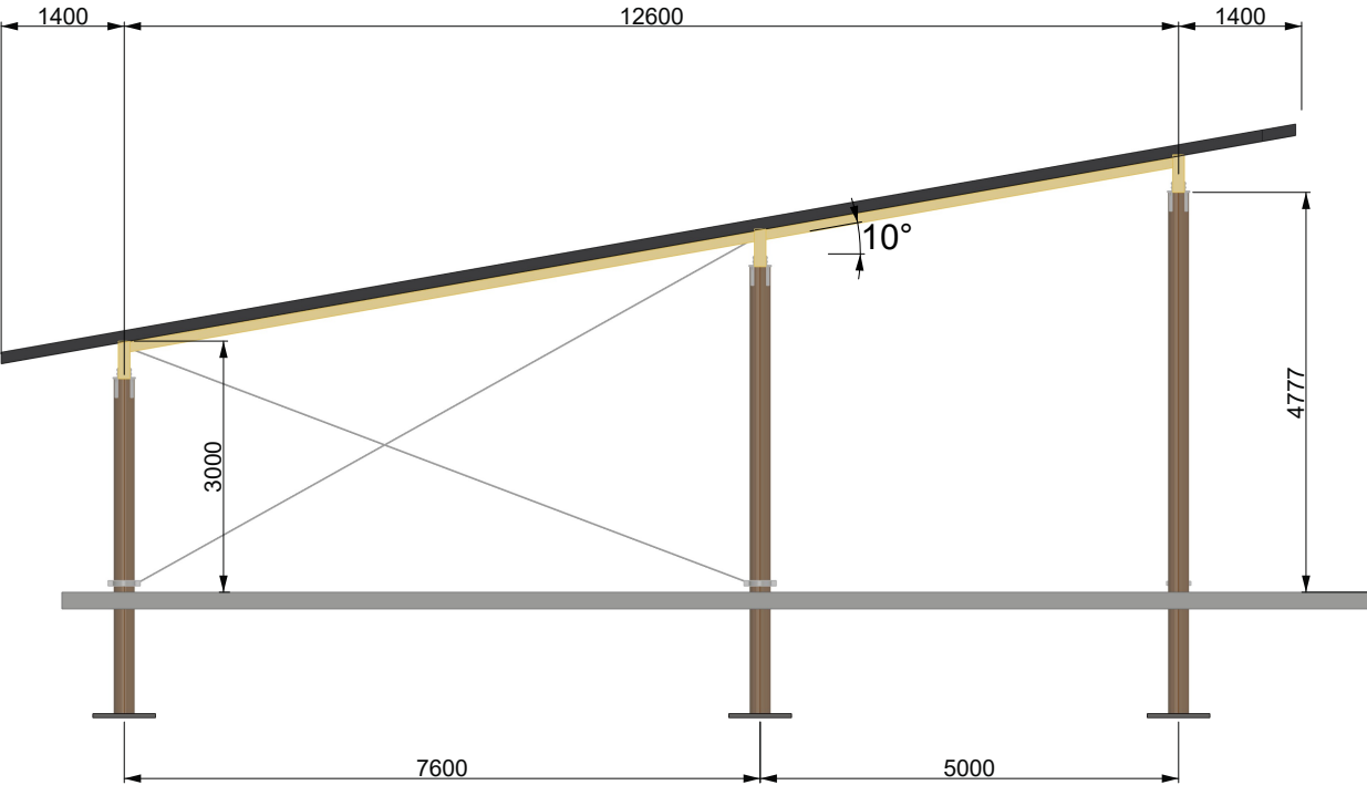
SEKTION GAVEL SKALA 1:100
