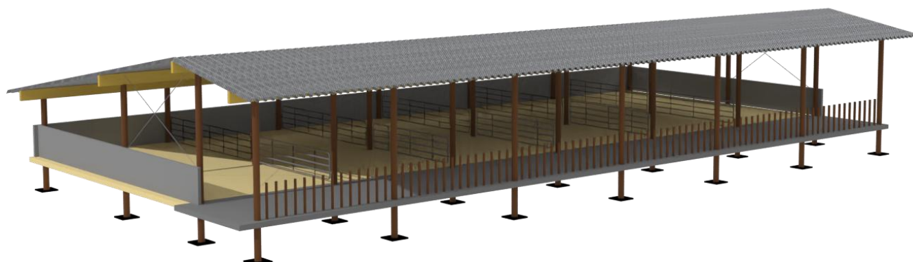
E - DJURSTALL, ASYMMETERISKT SADELTAK
