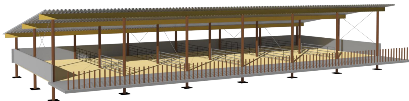
E - DJURSTALL, ASYMMETERISKT SADELTAK
