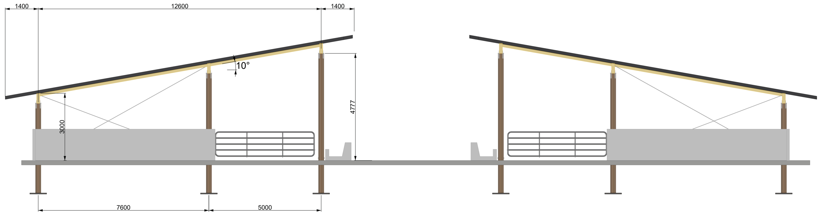
SEKTION GAVEL SKALA 1:100
